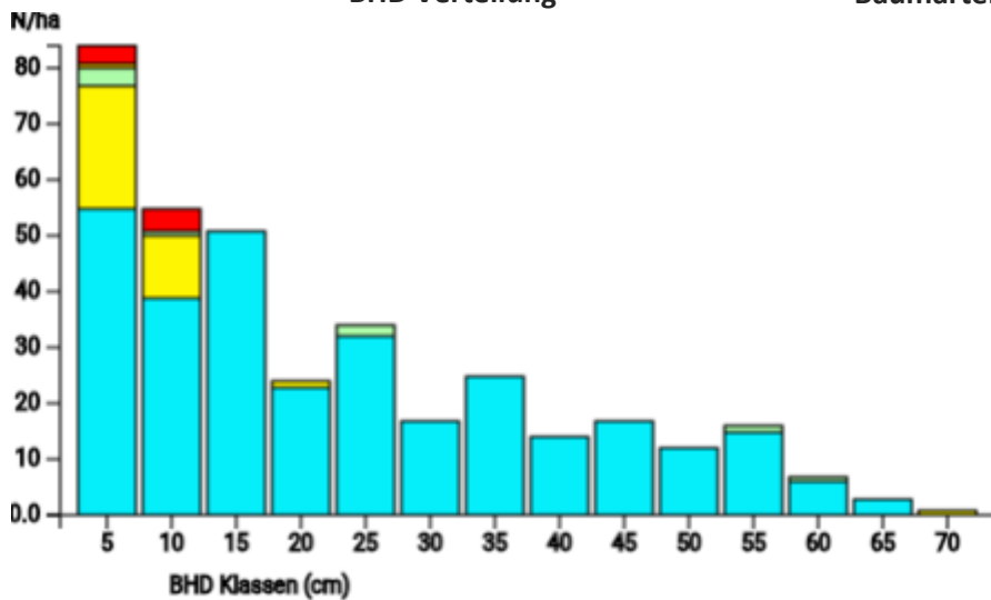
BHD Verteilung
